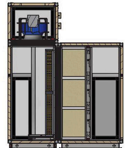
A-A (1 : 32)
